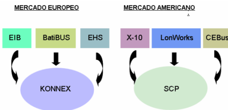
Figura 10. Plataformas de convergencia
