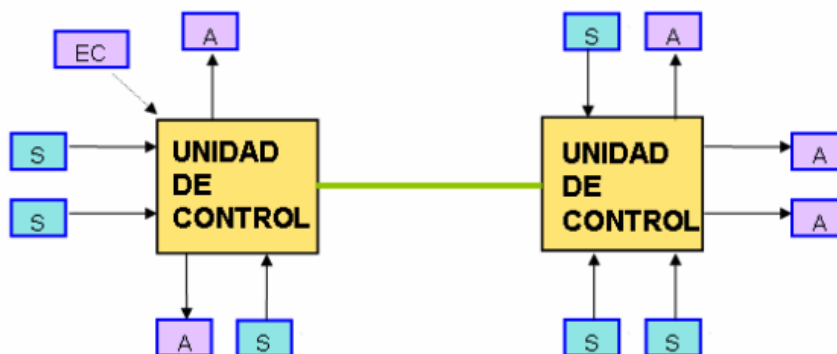
Figura 7. Esquema de arquitectura distribuida.
