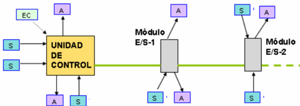
Figura 8. Esquema de arquitectura con periferia descentralizada
